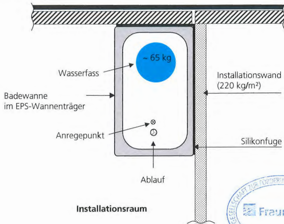
Lage des Prüfaufbaus im Installationsraum (EG vorne).
