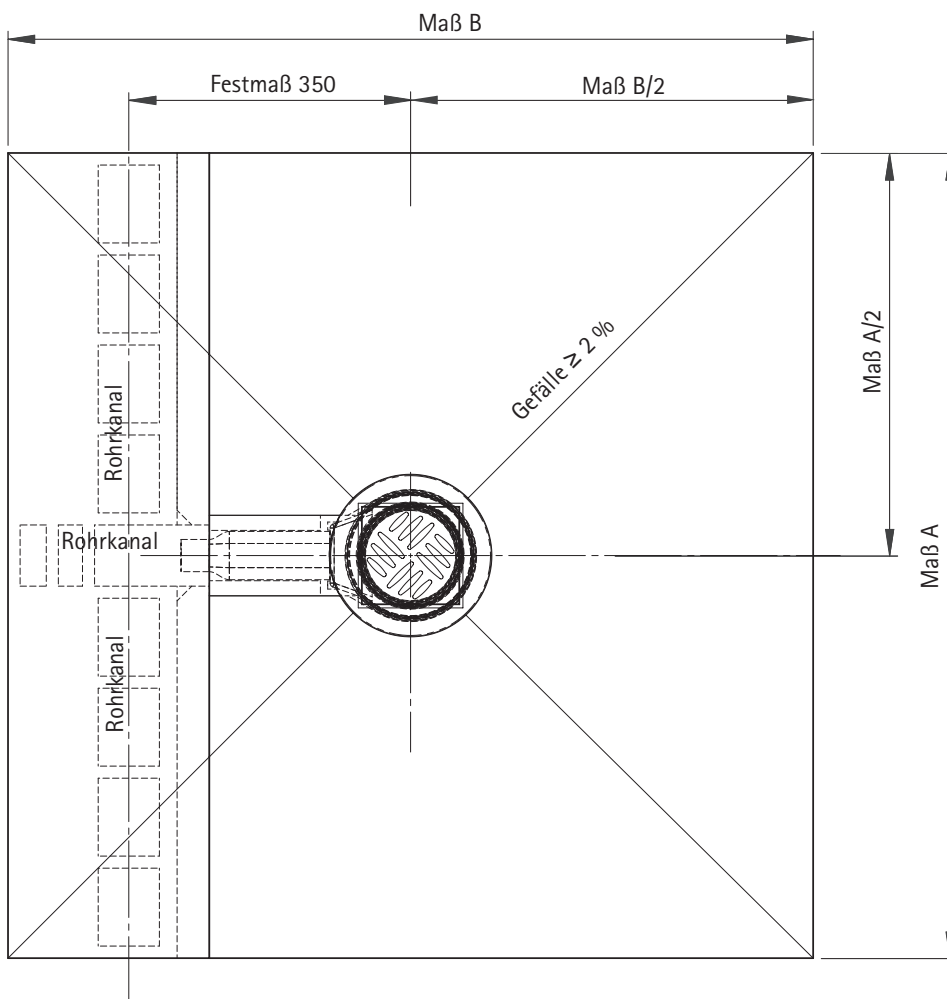
Draufsicht
