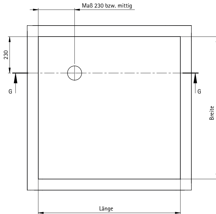
Draufsicht
