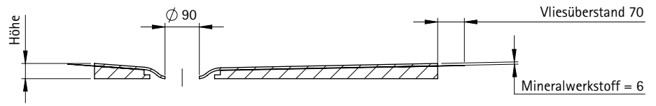
Schnitt G-G
