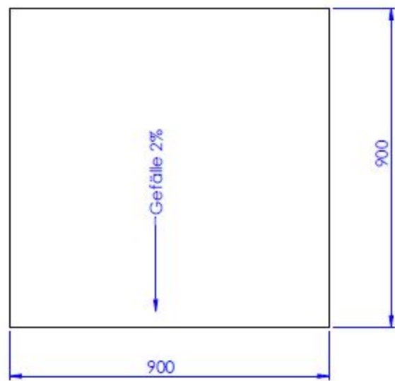
Draufsicht
