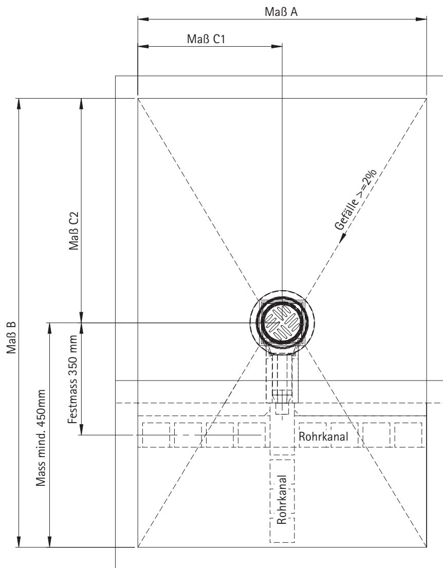
Allgemeine Draufsicht FLAT N
