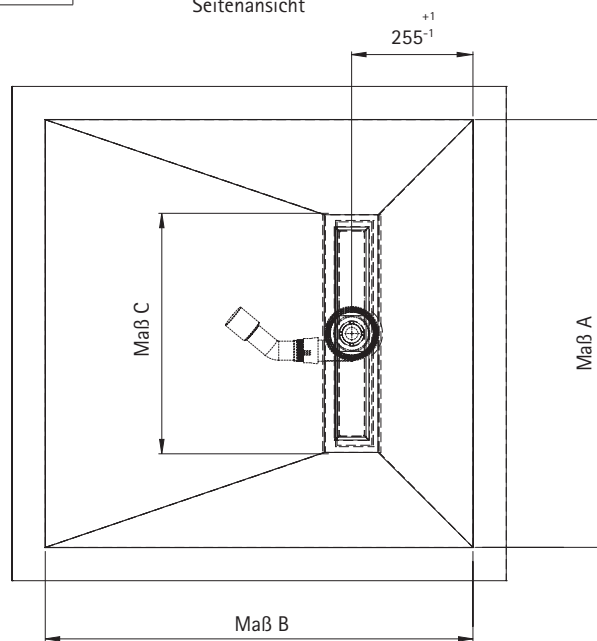
Allgemeine Draufsicht LINE PLUS PURE 4
