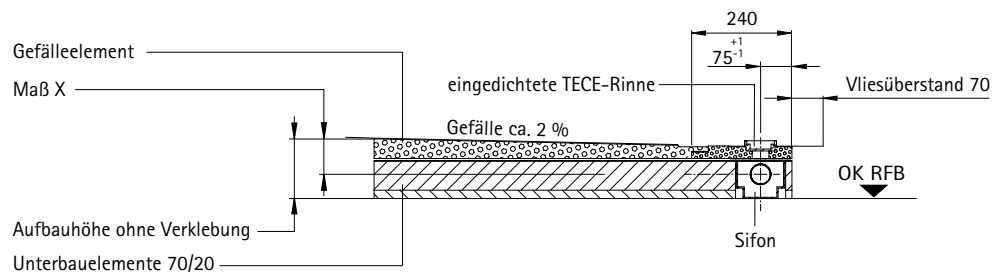
Schnitt A-A
