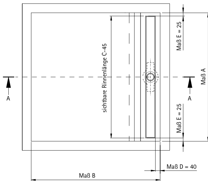
Allgemeine Draufsicht LINE2T
